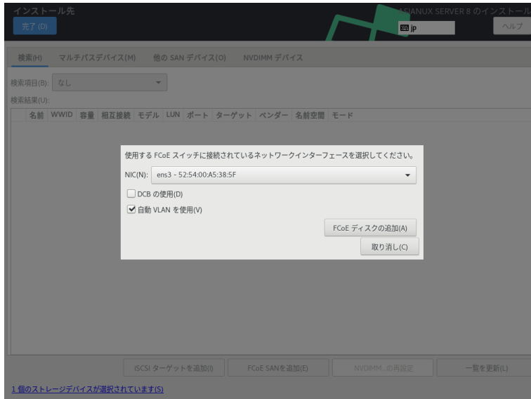
図 4-20 FCoE の追加
