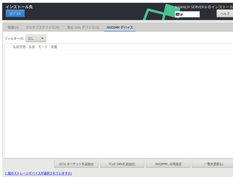
図 4-21 NVDIMM の追加
