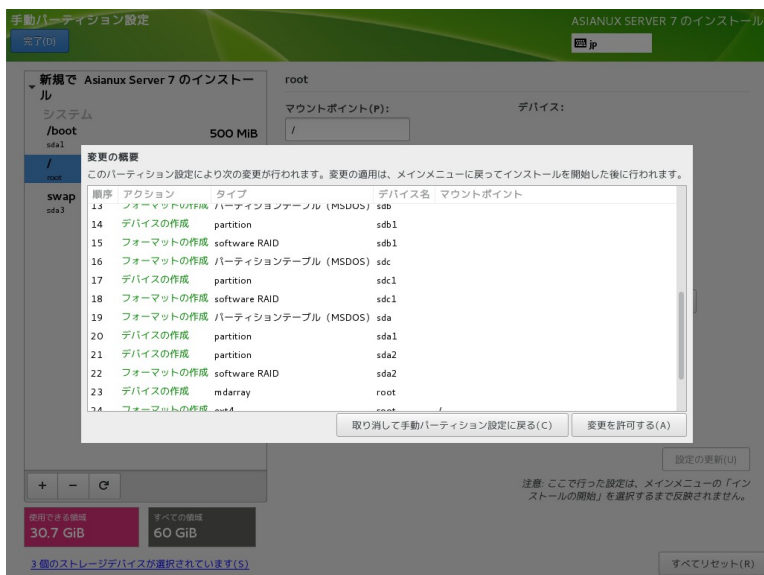
図 4-32 「完了(D)」をクリックした後の「変更の概要」の画面
