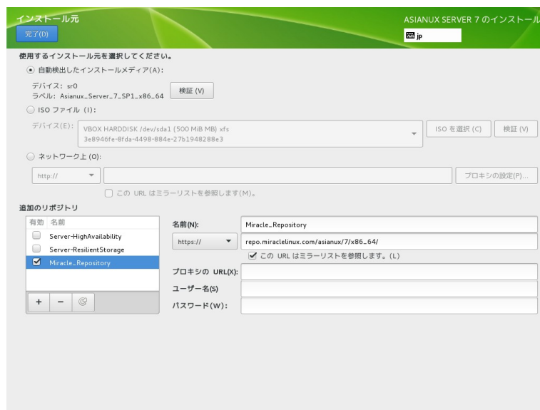
図 4-10 インストール元の選択
