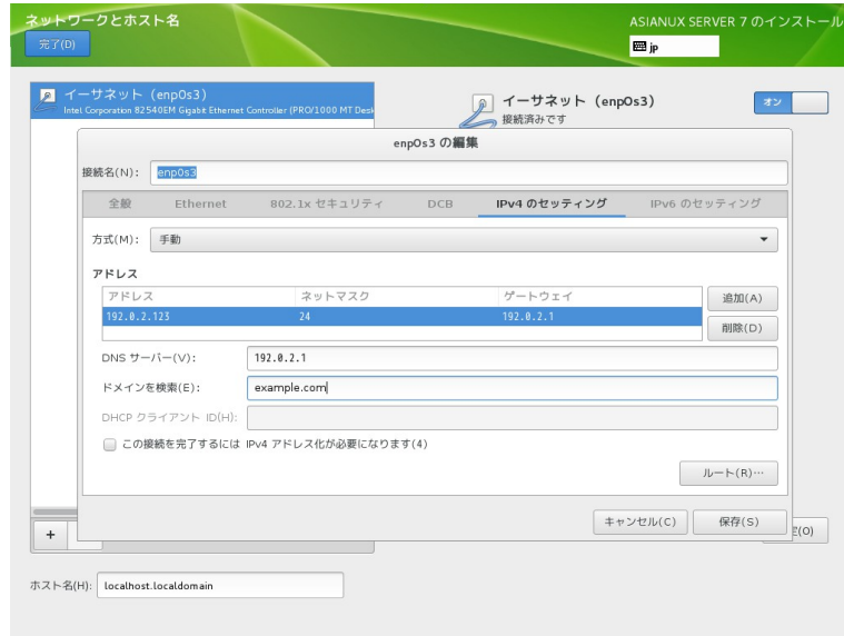
図 4-36 IPv4 手動設定
