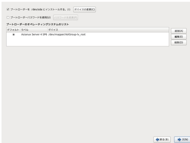
図 4-27 ブートローダー
