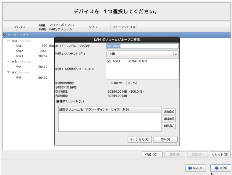
図 4-23 論理ボリューム作成
