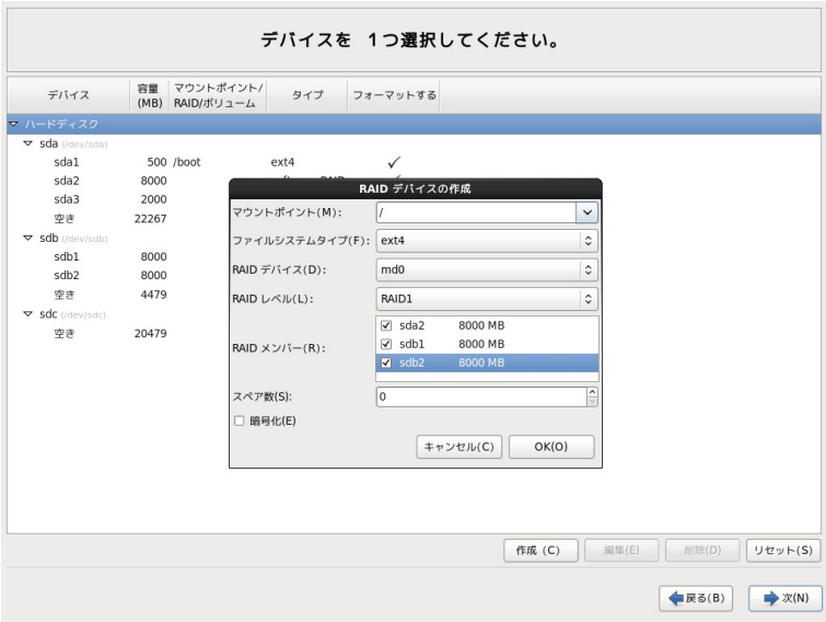
図 4-19 RAID デバイスの構成
