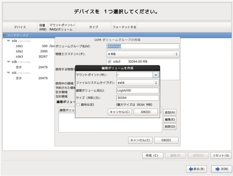
図 4-24 マウントポイント指定
