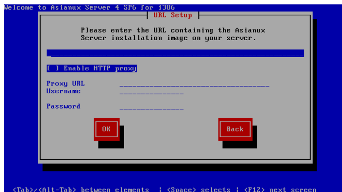
図 3-6 FTP, HTTP の設定
