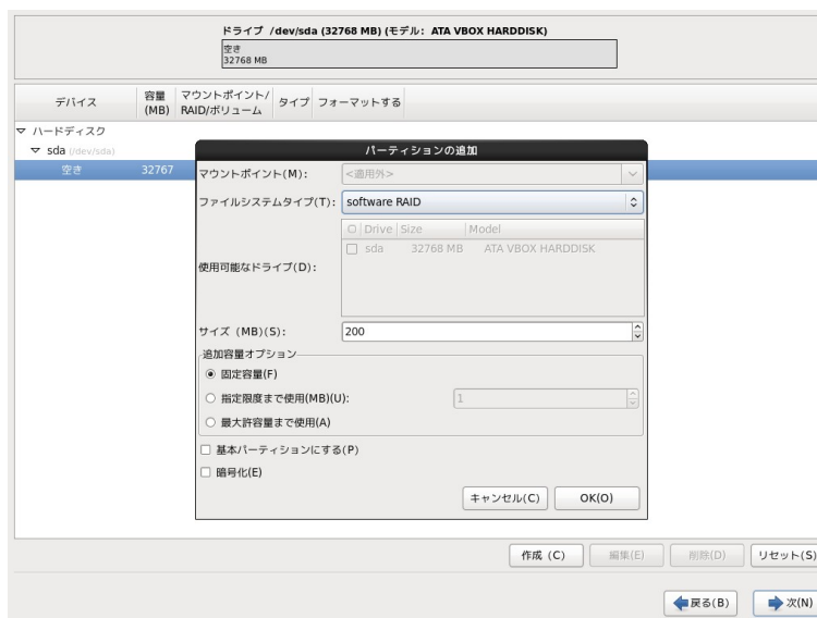
図 4-17 ソフトウェア RAID パーティション作成
