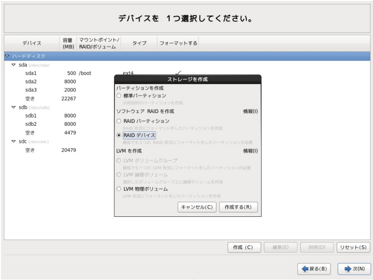
図 4-18 RAID デバイス作成画面
