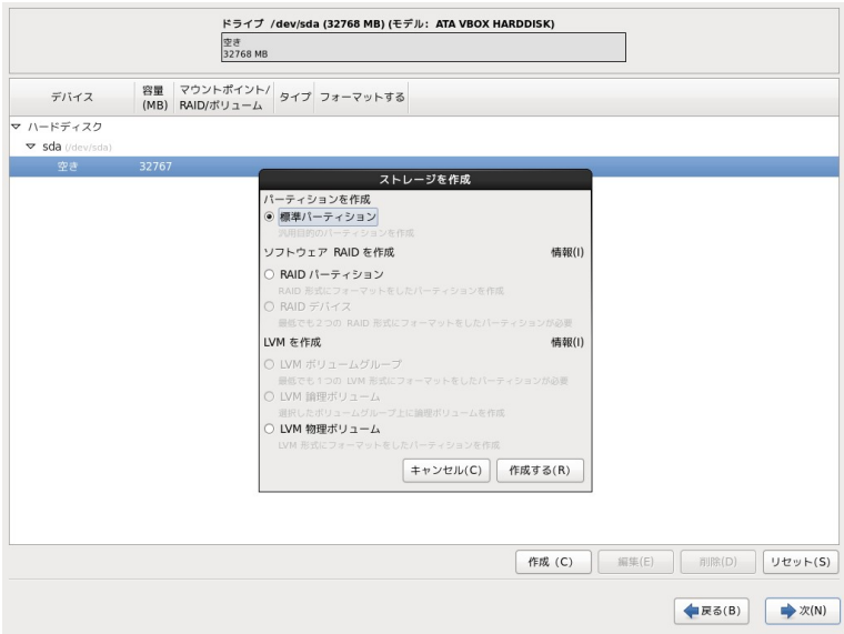
図 4-14 パーティション新規作成
