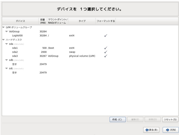
図 4-26 LVM パーティション作成例
