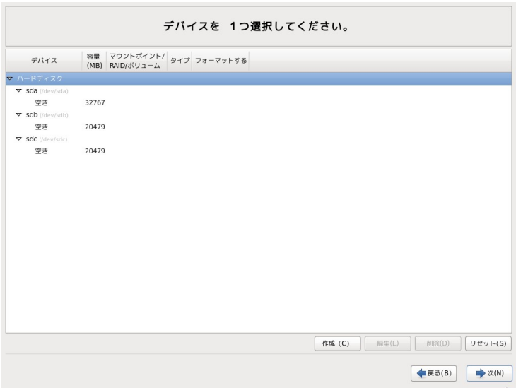
図 4-13 パーティションの手動設定画面
