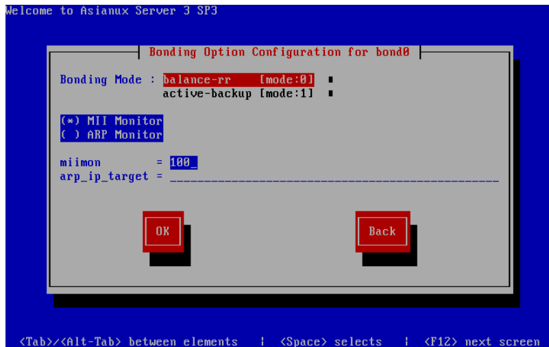
図 5-25 ボンディングモード設定
