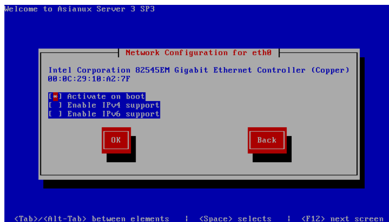
図 5-16 ネットワーク設定
