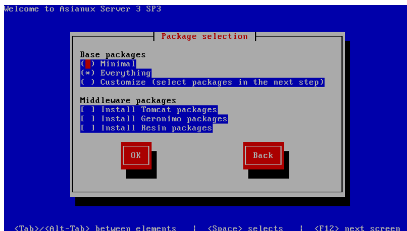
図 5-28 パッケージ選択
