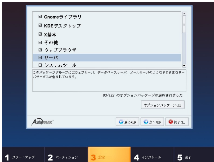
図 4-28 パッケージのカスタマイズ
