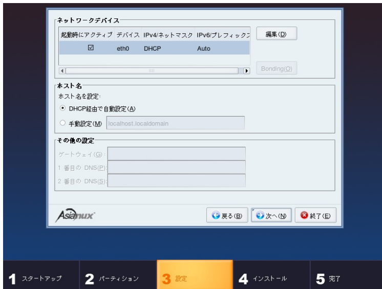
図 4-20 ネットワーク
