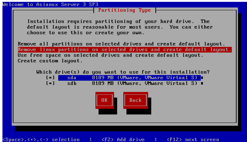
図 5-6 自動パーティション設定
