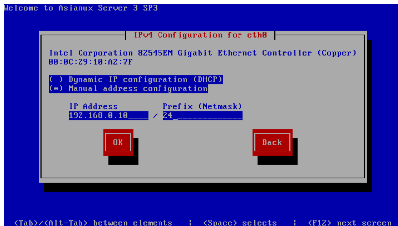
図 5-17 IPアドレス設定
