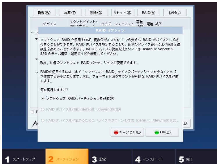
図 4-9 ソフトウェア RAID パーティション作成
