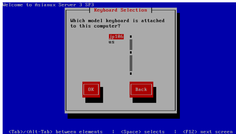
図 5-5 キーボード設定
