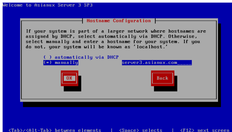
図 5-19 ホスト名設定
