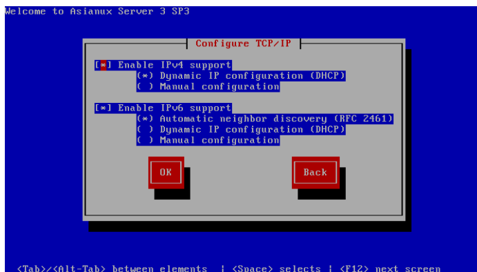
図 3-4 TCP/IP 設定
