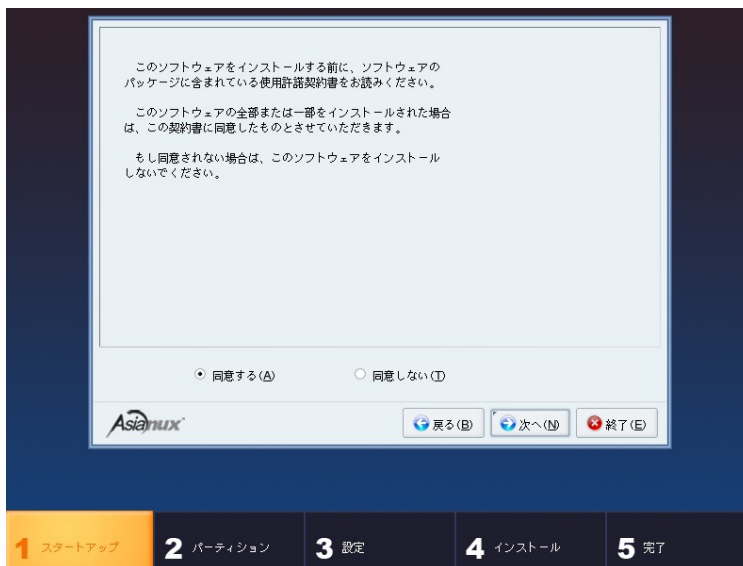
図 4-3 使用権許諾
