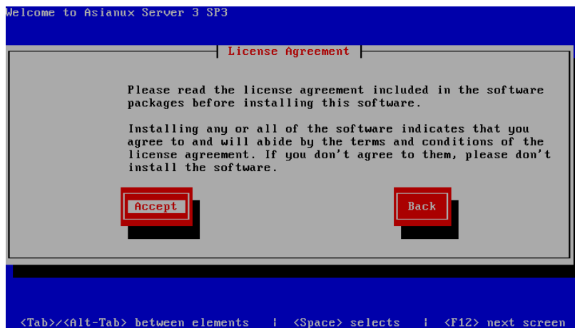
図 5-4 使用権許諾
