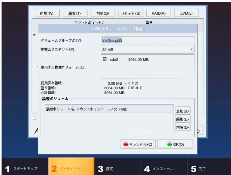
図 4-16 ボリュームグループ作成画面
