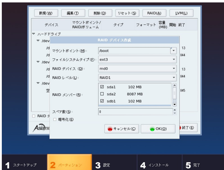
図 4-12 RAID デバイス作成画面
