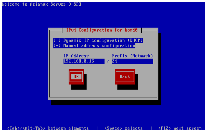
図 5-24 ボンディング IP アドレス設定
