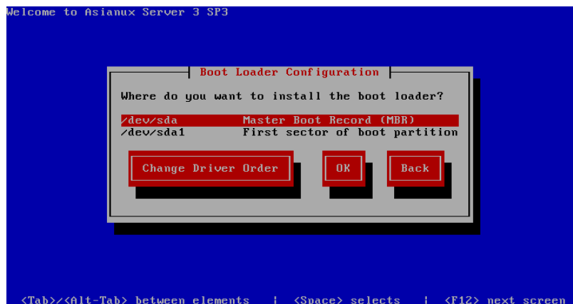
図 5-14 ブートローダのインストール先の設定
