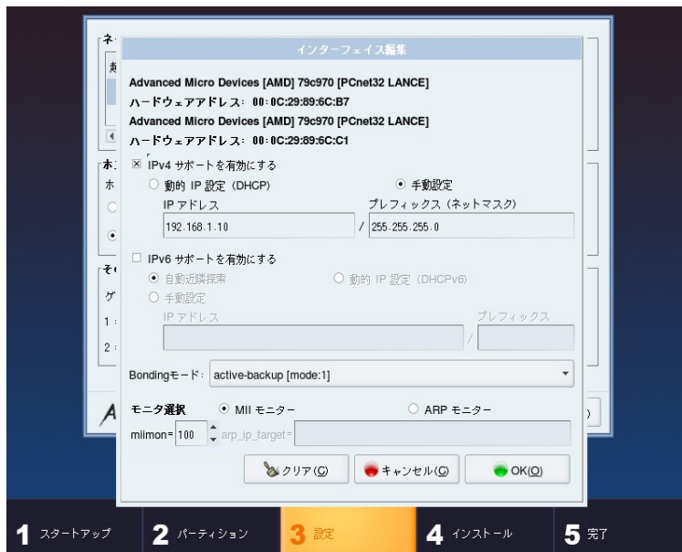
図 4-24 ボンディングインターフェイスの設定
