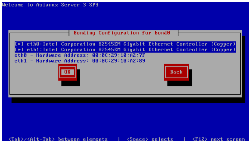
図 5-21 ボンディングインターフェイス設定
