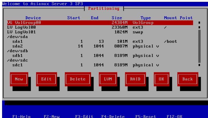
図 5-9 パーティションの手動設定
