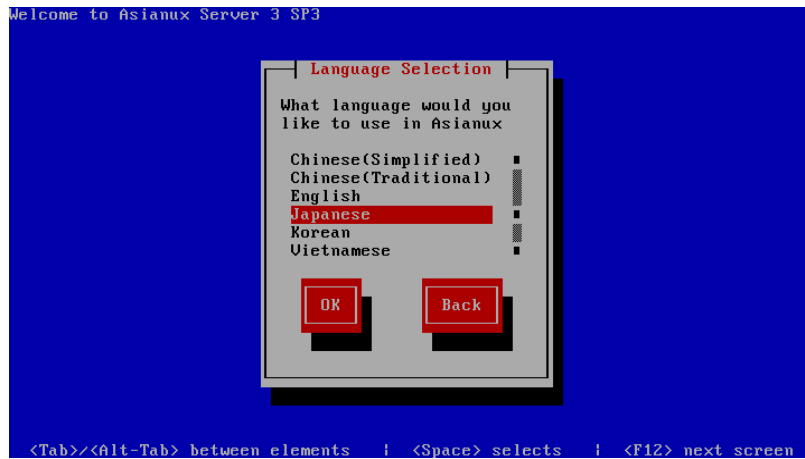
図 5-2 言語選択
