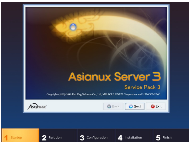
図 4-1 スタート
