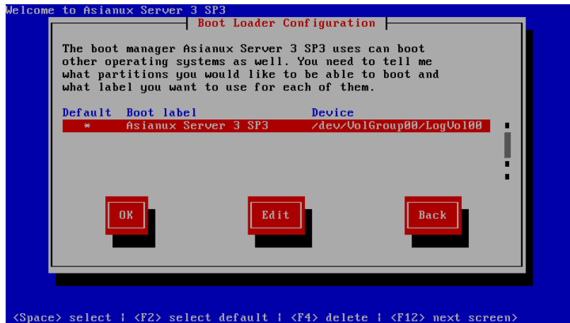
図 5-13 ブートローダ設定
