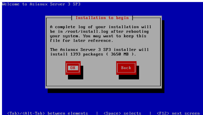
図 5-30 インストール確認
