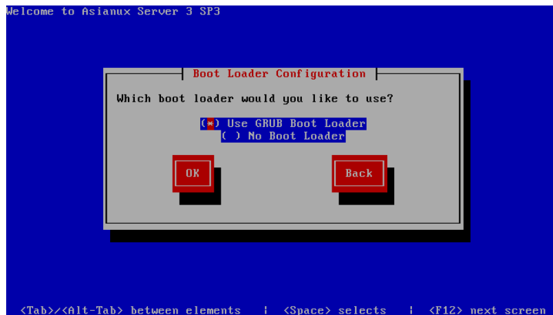
図 5-10 ブートローダ設定
